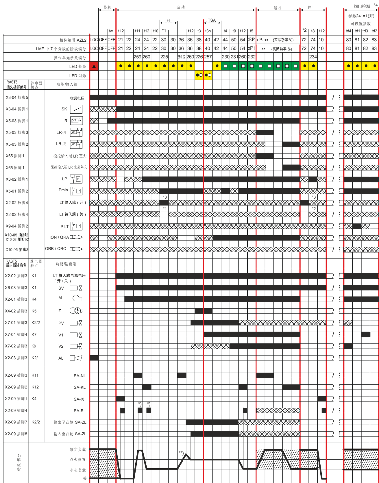
插图 4: 燃料管路 G 的程序进程不带或带阀门检漏, Gp1 带阀门检漏和 Gp2 不带阀门检漏
