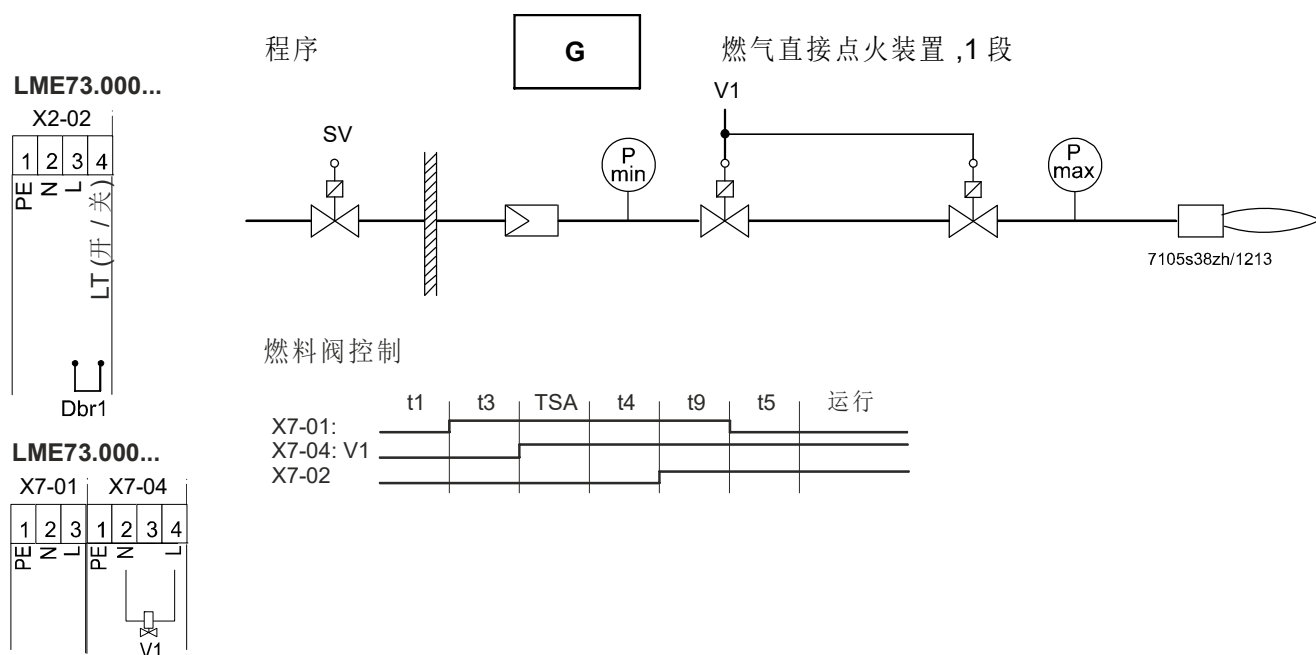
插图 5: 燃气直接点火装置 (G) 燃料管路, 1 段, 不带阀门检漏
