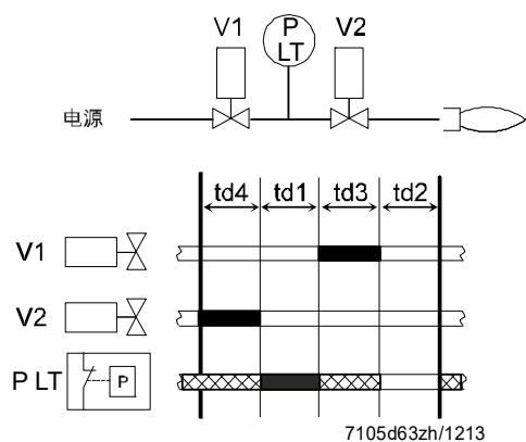
插图 9: 利用独立的压力开关进行阀门检漏
