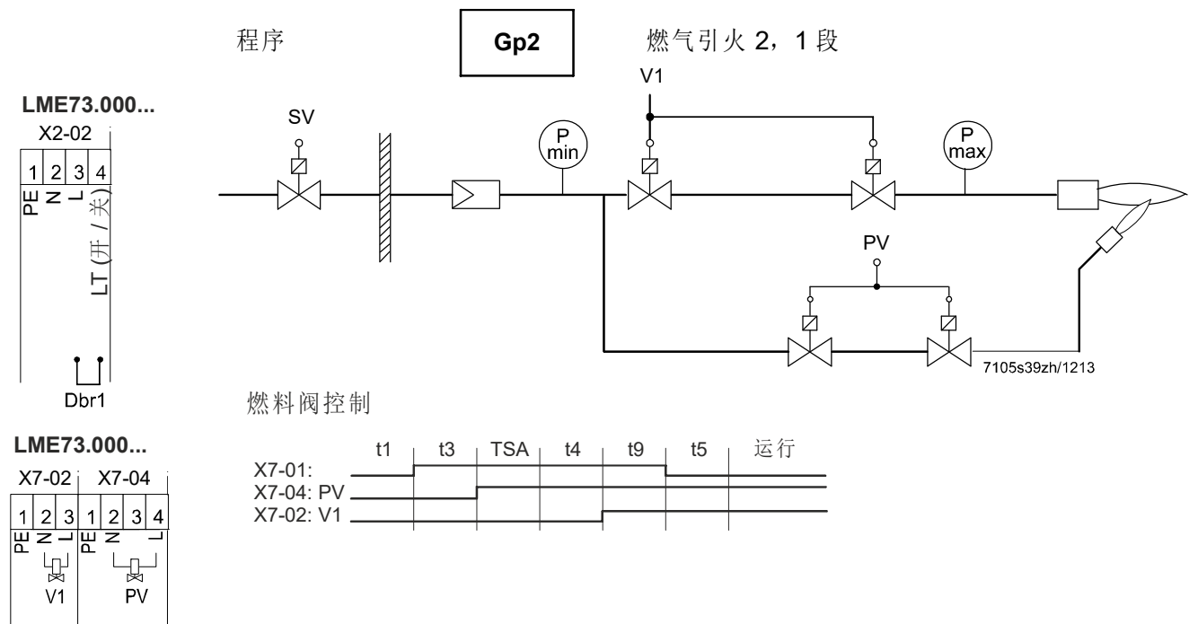
插图 8: 燃气引火 2 (Gp2) 燃料管路, 1 段, 不带阀门检漏
