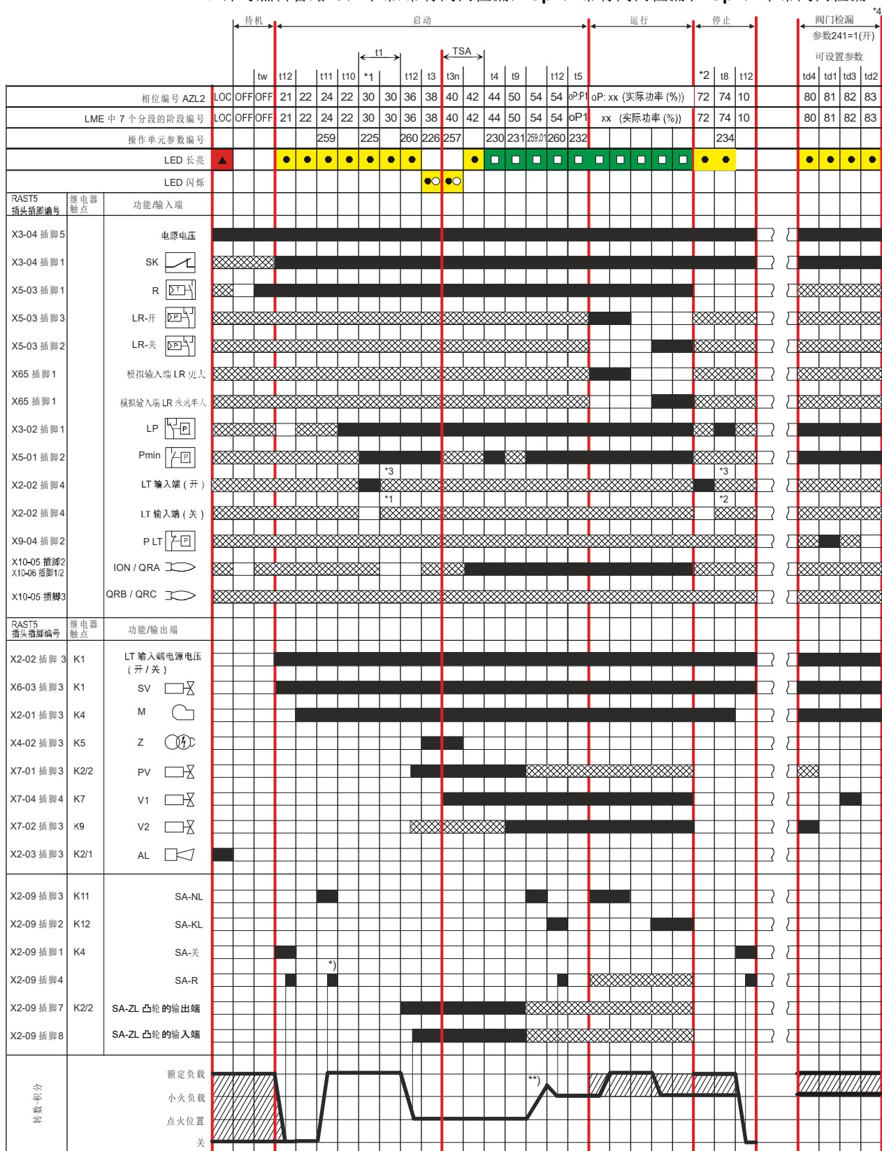
插图 1: 燃料管路 G 的程序进程不带或带阀门检漏， Gp1 带阀门检漏和 Gp2 不带阀门检漏
