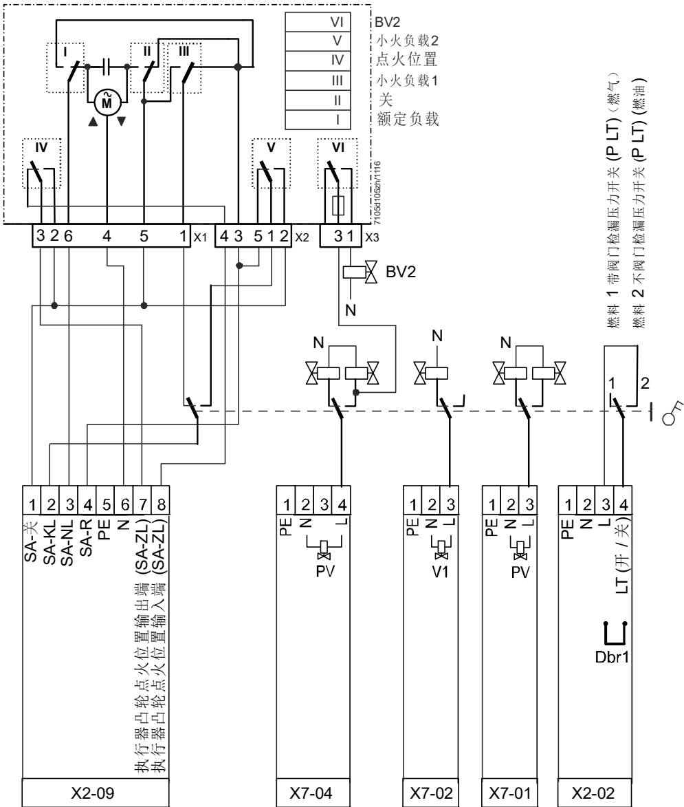
插图12: 带执行器 SQM4 的 LME73.000Ax 连接图 (范例 3)
