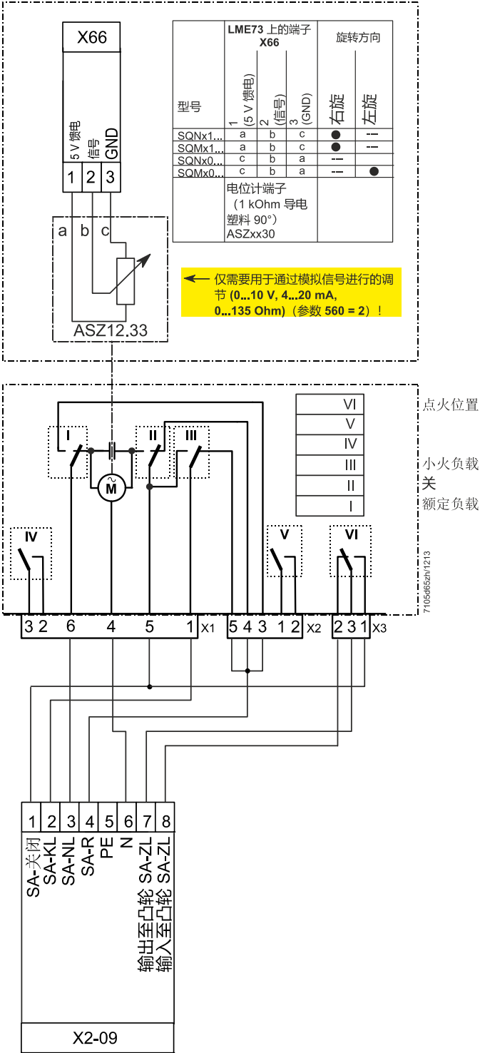
插图 10: 带执行器 SQM4 的 LME73.000Ax 连接图 (范例 1)
