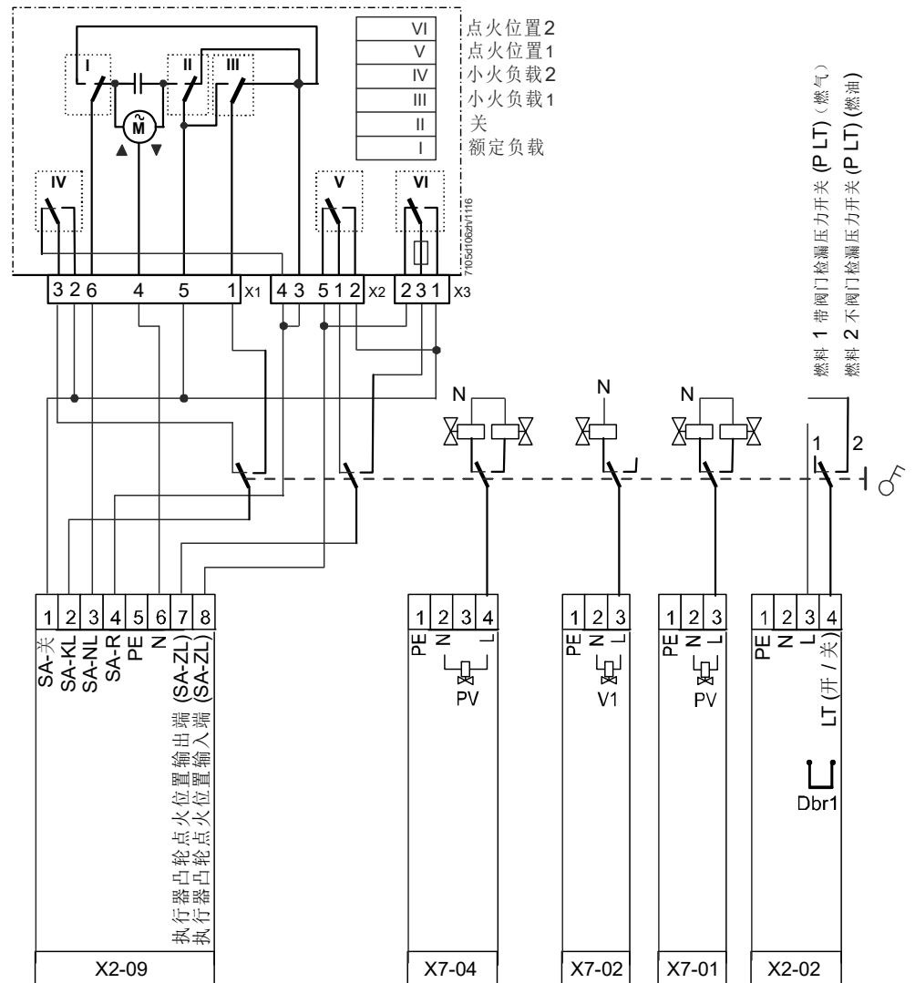
插图13: 带执行器 SQM4 的 LME73.000Ax 连接图 (范例 4)
