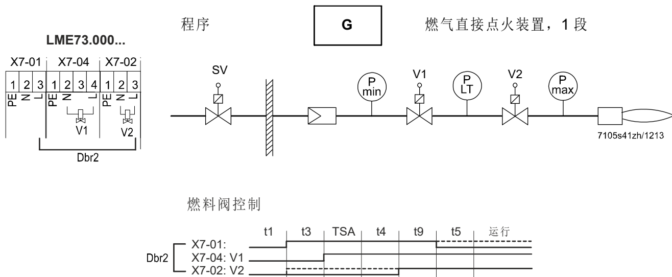
插图 6: 燃气直接点火装置 (G) 燃料管路, 1 段, 带阀门检漏
