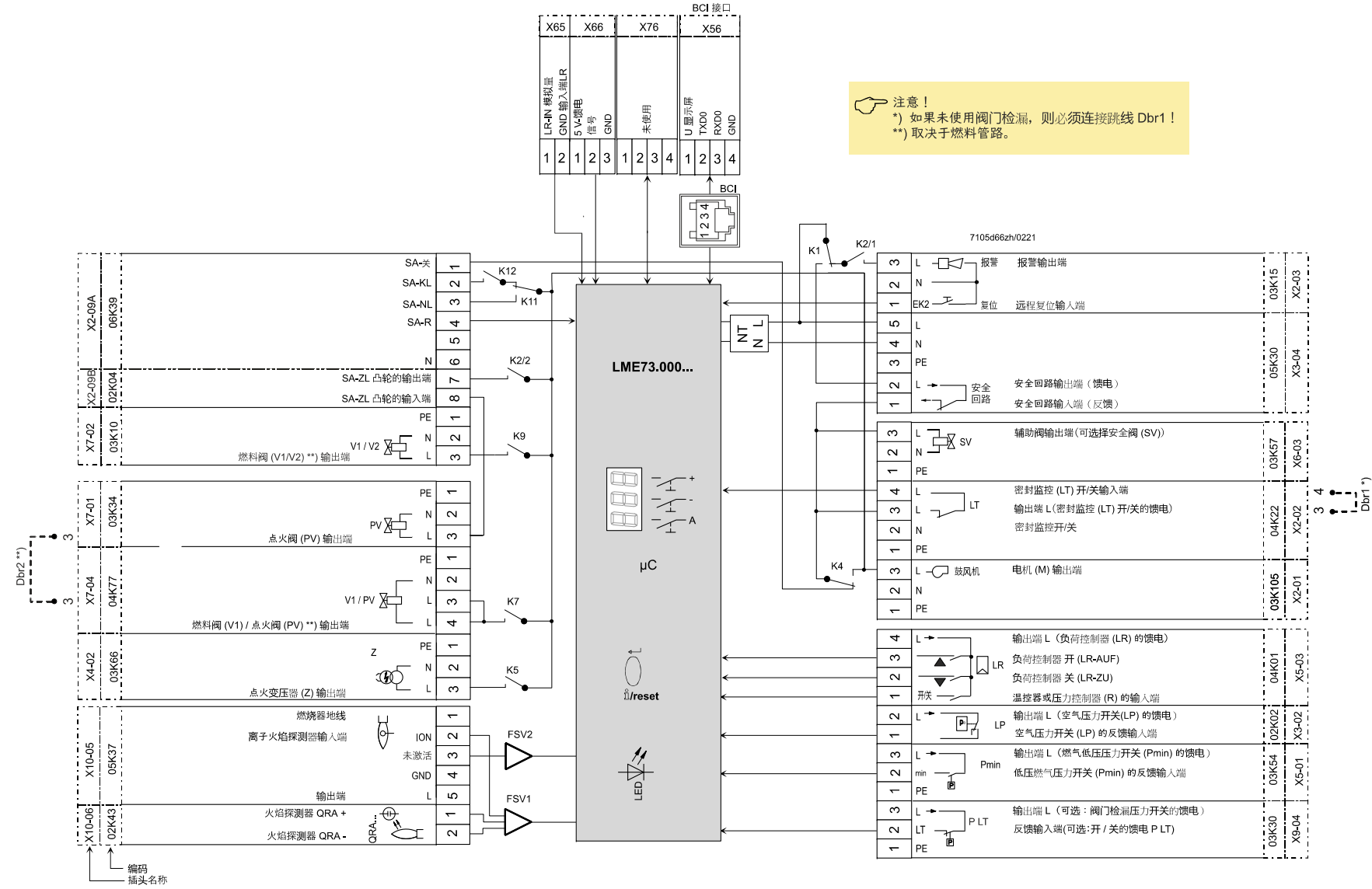
插图 14: 输入和输出/内部连线图
