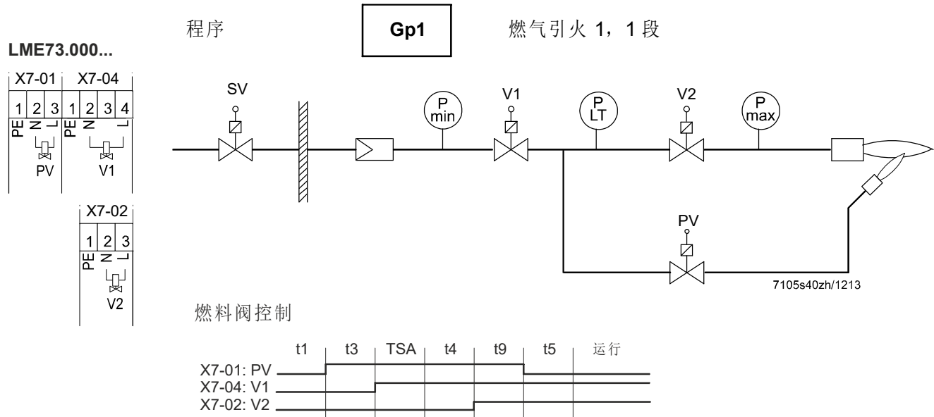
插图 7: 燃气引火 1 (Gp1) 燃料管路, 1 段, 带阀门检漏, 交替燃烧的点火燃烧器
