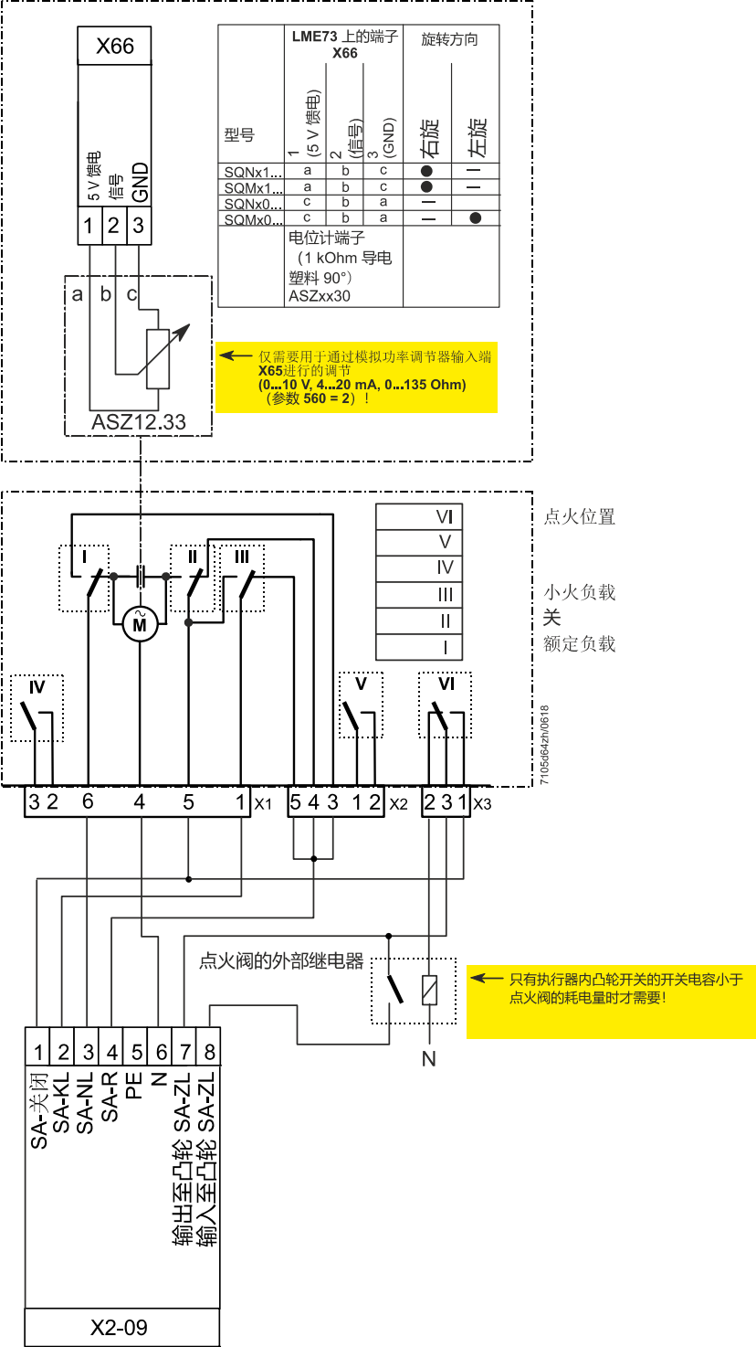
插图 11:带执行器 SQM4 的 LME73.000Ax 连接图 (范例 2)
