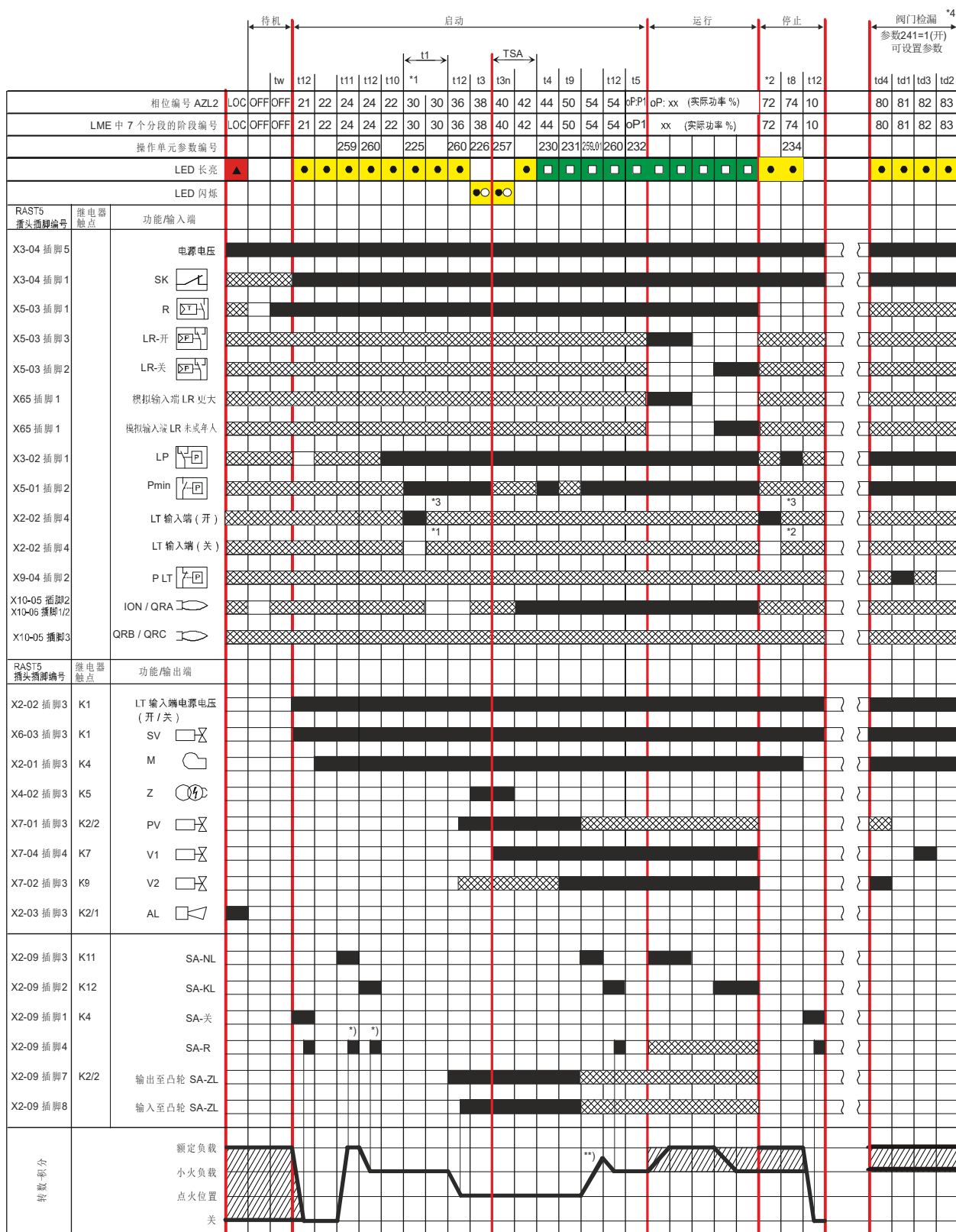
插图 3: 燃料管路 G 的程序进程不带或带阀门检漏, Gp1 带阀门检漏和 Gp2 不带阀门检漏
