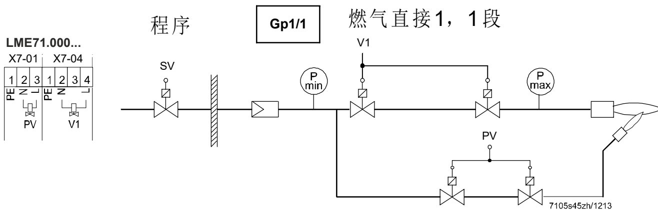
插图 3: 燃料管路燃气引火 1 (Gp1/1)，1 段
