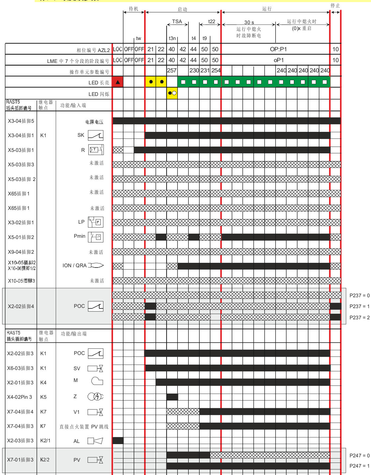
插图 1: 燃料管路 G 和 Gp1/1 的程序进程
