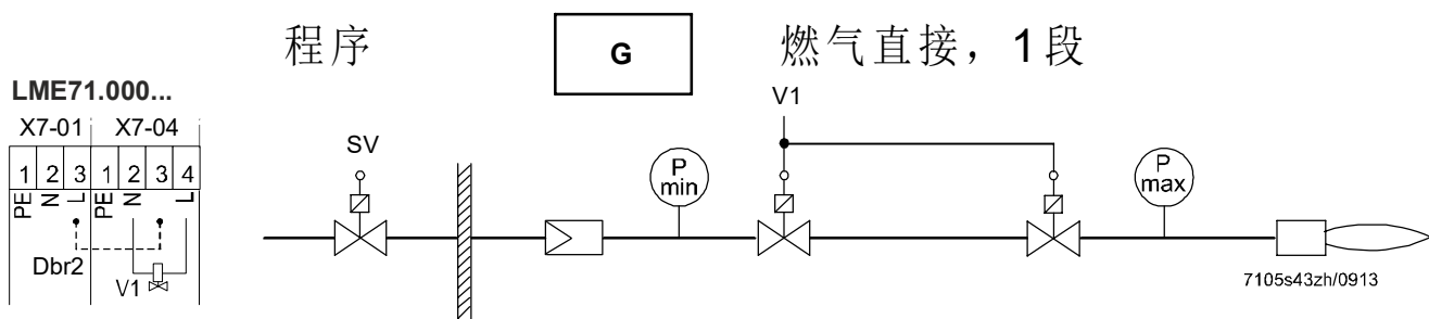
插图 2: 燃油管路燃气直接点火 (G)，1 段
