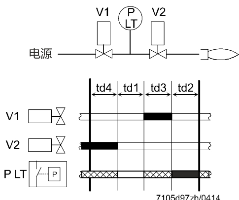
图 4: 配备独立燃气压力开关的阀门检漏
