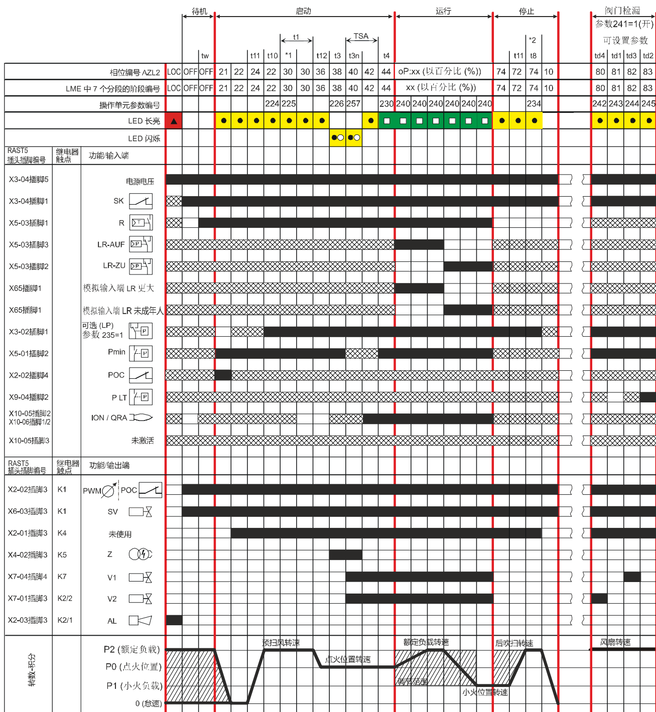
图 1: 无/有阀门检漏功能的燃料管路 G 的程序进程
