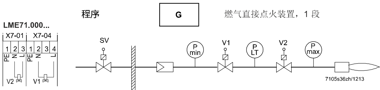
图 3: 燃料管路燃气直接点火 (G)，1 段,有阀门检漏
