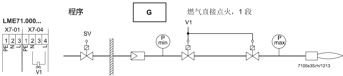
图 2: 燃料管路燃气直接点火 (G)，1 段
